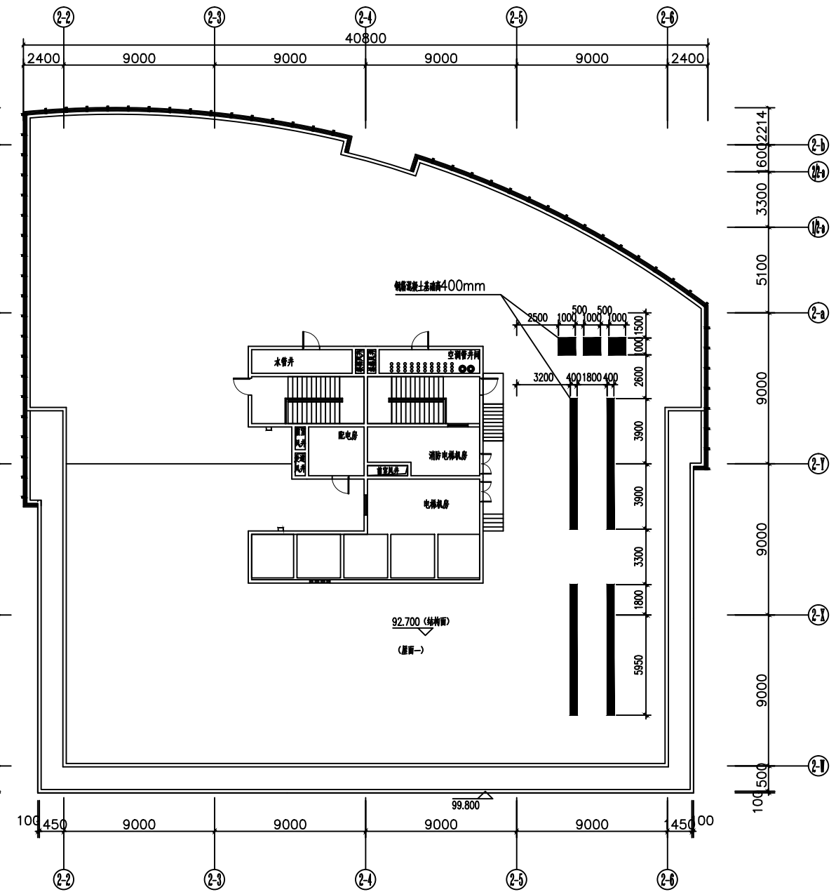
B-2 屋面风冷热泵系统设备基础平面图 1:150
