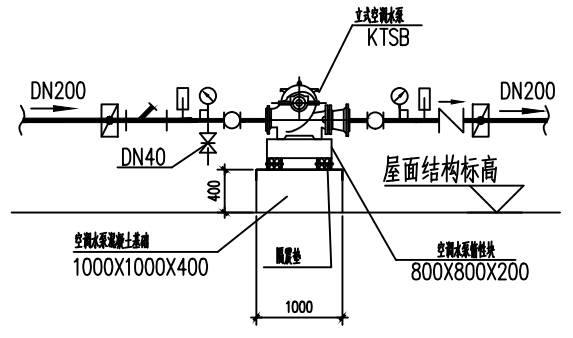
立式空调水泵安装示意图
