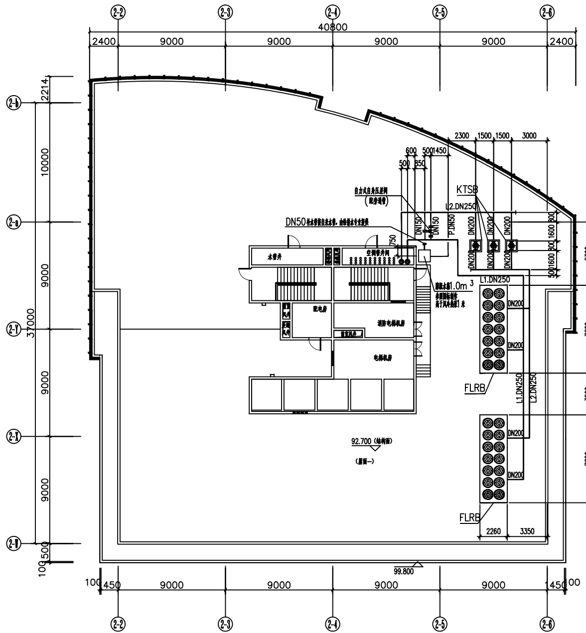
B-2 屋面风冷热泵系统设备平面图 1:150
